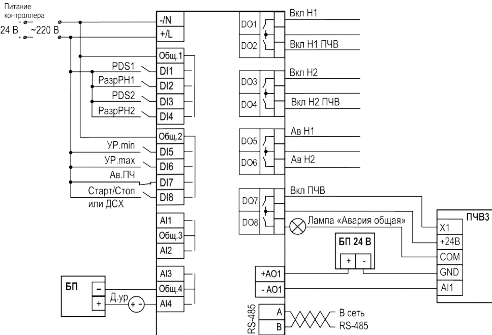
Рисунок 5.8 – Схема подключения
