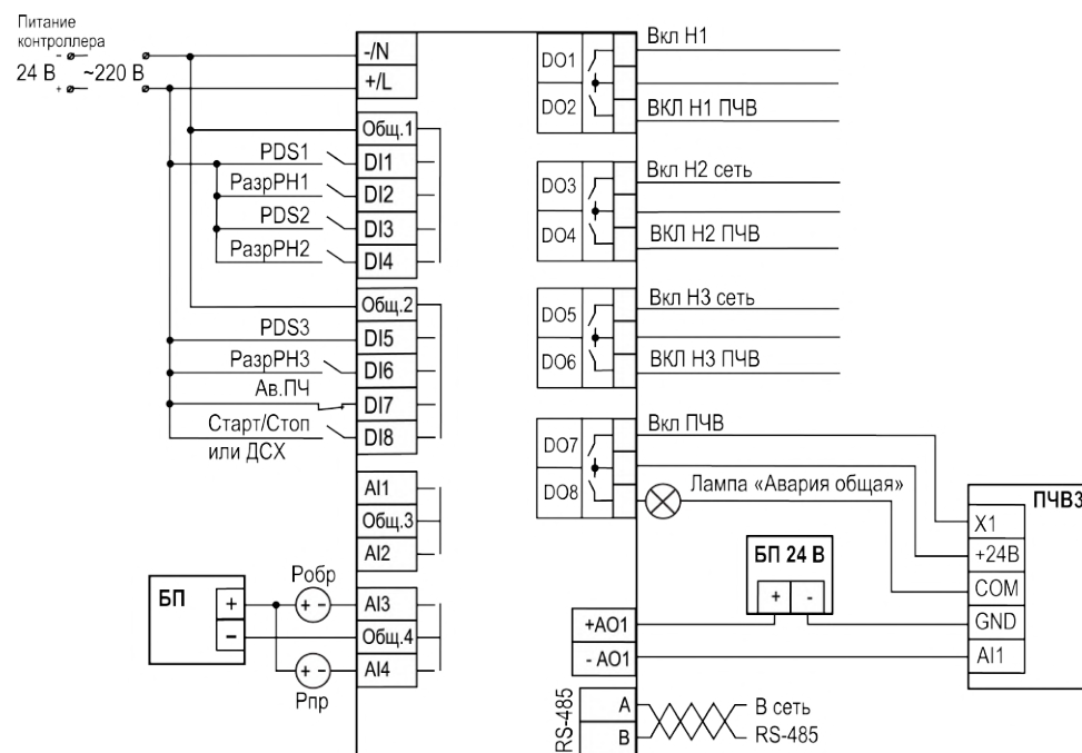
Рисунок 5.7 – Схема подключения
